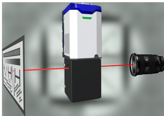
事例： カメラレンズとテストチャートの平行出し
